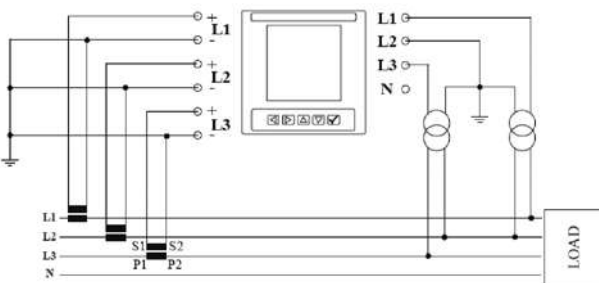
Подключение через 3 ТТ и 2 ТН
