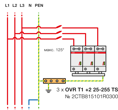
Конфигурация 2 7 \text{ кА} \leq I_p \leq 15 \text{ кА}
