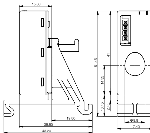
Датчик (CMS-200DR)
