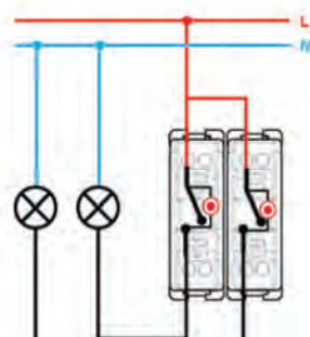
Выключатель двухклавишный с подсветкой
