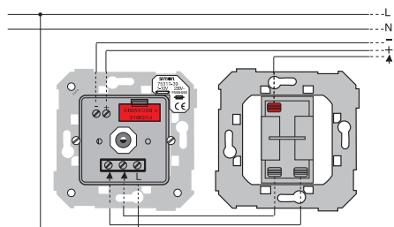
Светорегулятор и переключатель проходной
