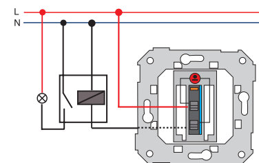
Подключение при помощи реле
