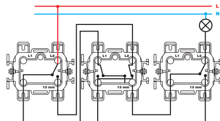
Выключатель перекрёстный с 3-х мест 73201-39 + 73251-39 + 73201-39
