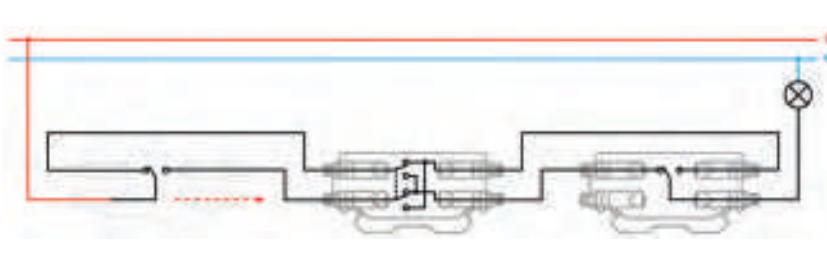
Переключатель перекрёстный (Cx.7)
