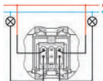
Выключатель карточный 2-полюсный
