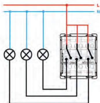
Выключатель трёхклавишный (Сх.05)
