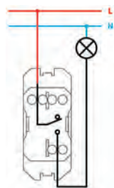
Однополюсный выключатель (Сх.1, Сх.1S)
