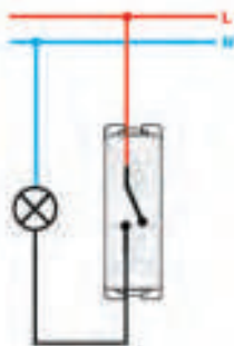
Однополюсный выключатель (Сх.1)
