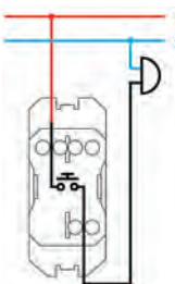
Кнопочные выключатели с НО-контактом
