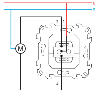
Трёхпозиционный выключатель жалюзи с фиксацией клавиши (Сх.4)
