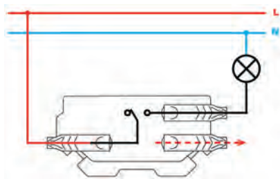
Однополюсный выключатель (Cx.1)
