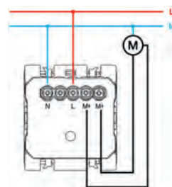
Выключатель жалюзи электронный
